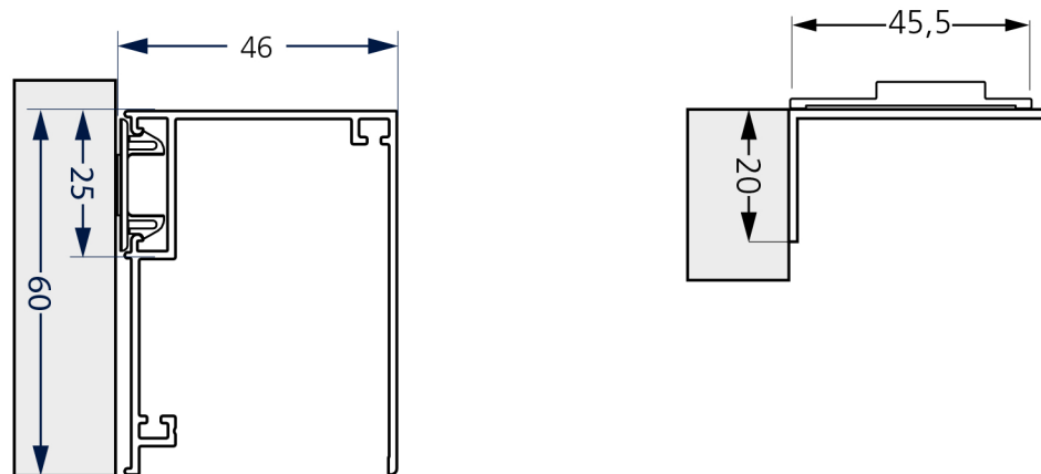
Montage bovengeleider en L-profiel
